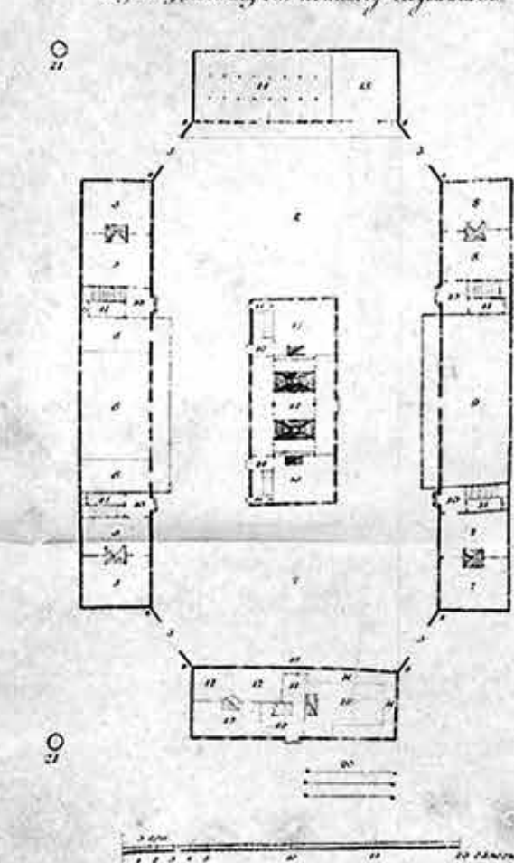
Начертание ПРЕДОХРАНИТЕЛЬНОГО ДОМА для жилищи кочану служивки.
